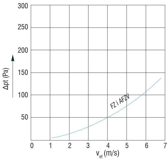
Dijagram pada tlaka FZ
