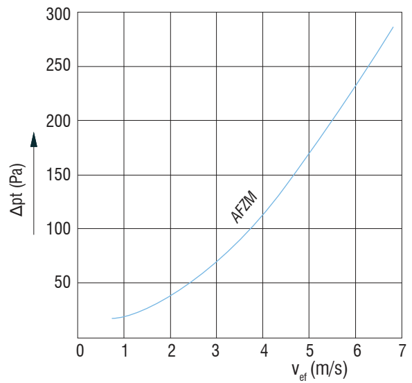
Dijagram pada tlaka AFZM, AFZV
